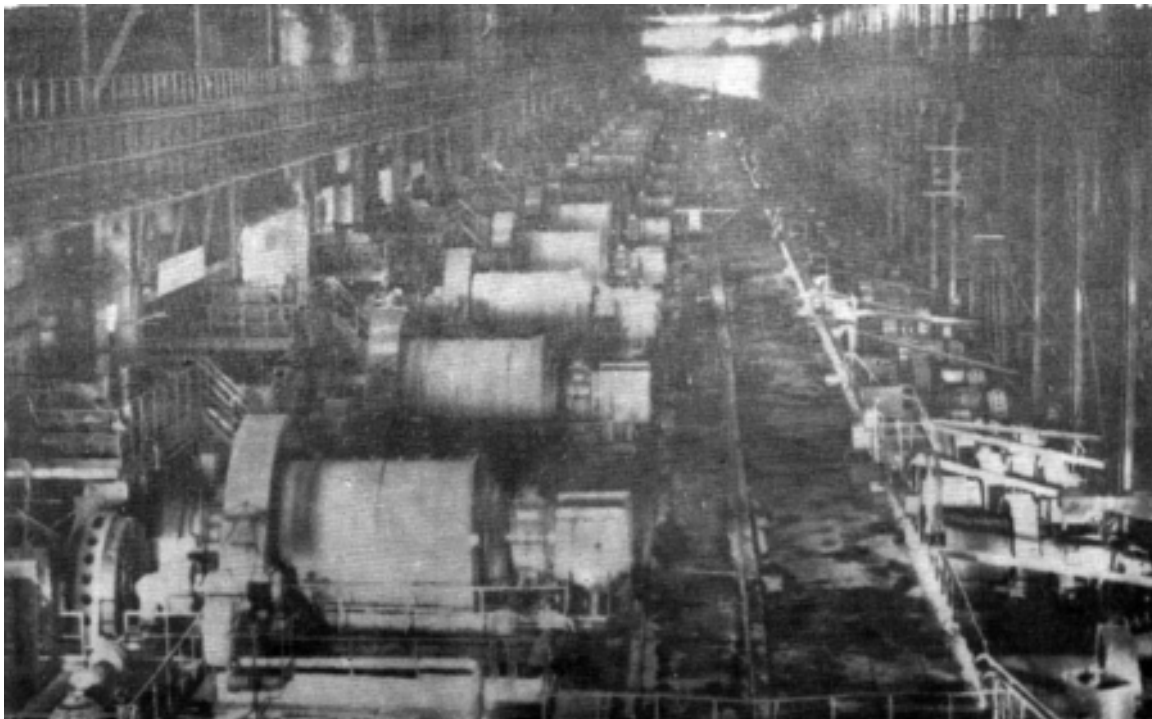
Сегодня на фабрике обогащения (мельничный пролет).
