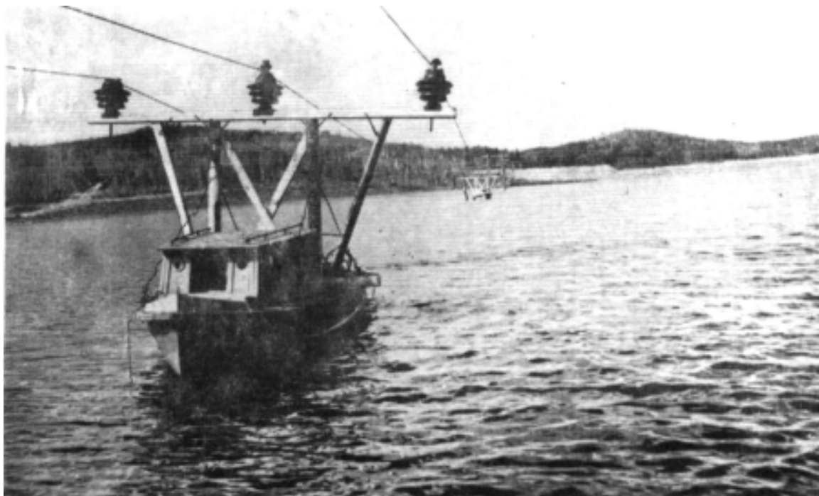
По временной схеме (высоковольтная ЛЭП, питающая фабрики комбината).
