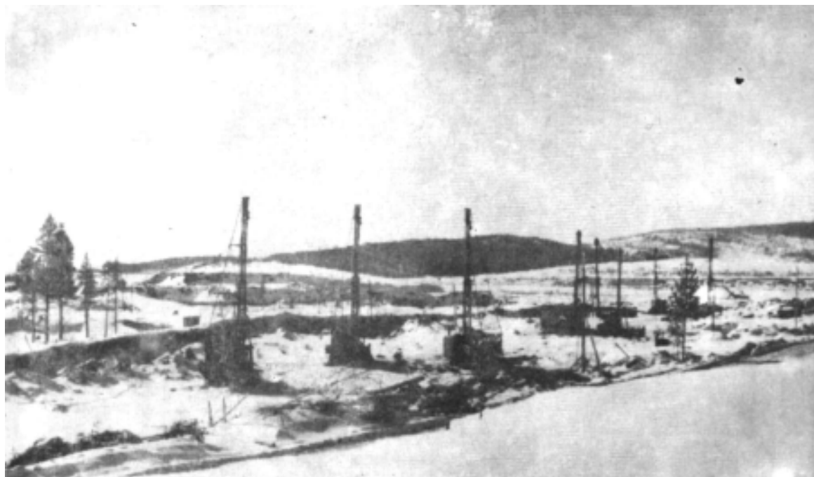
Главный карьер. Станки канатно-ударного бурения - первое поколение бурильных станков Качканарского ГОКа
