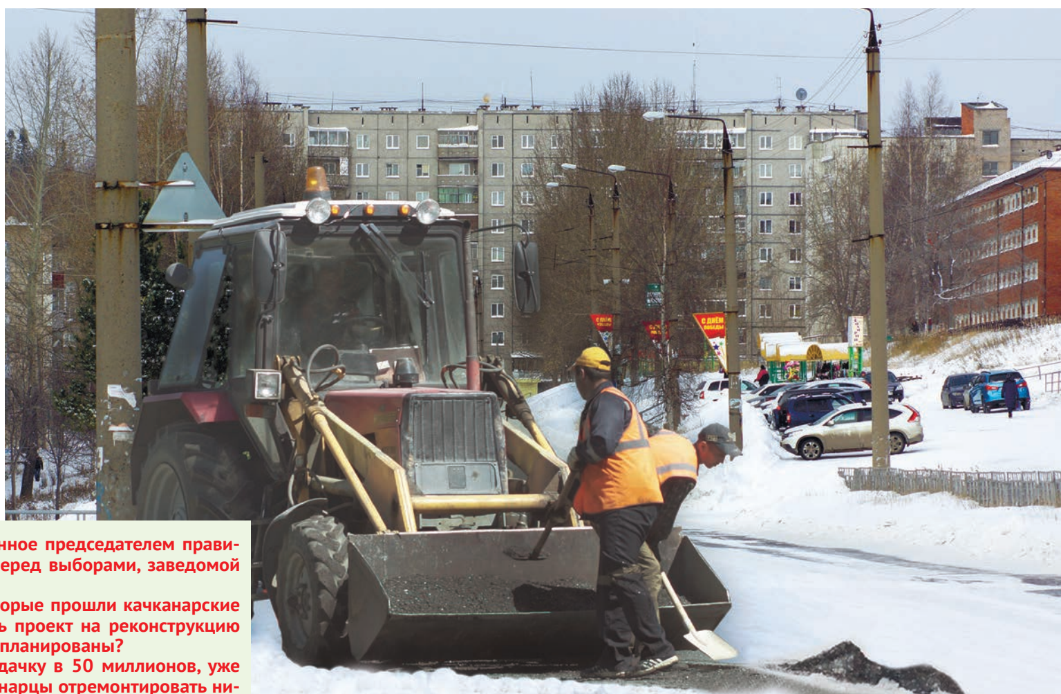
Реконструкция событий
